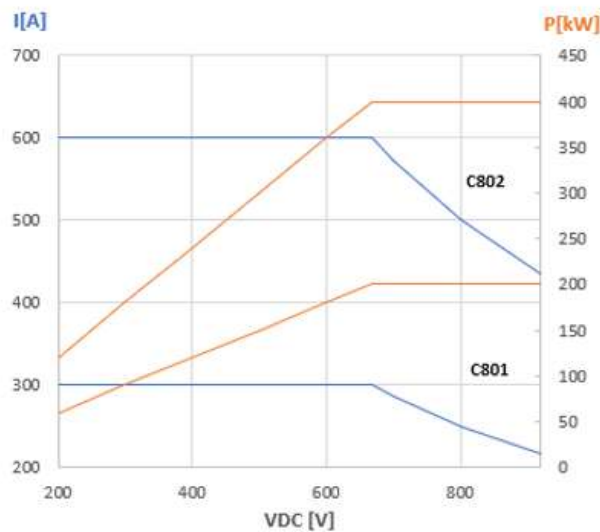
Figura 1. Curva di potenza (funzionamento standard)
